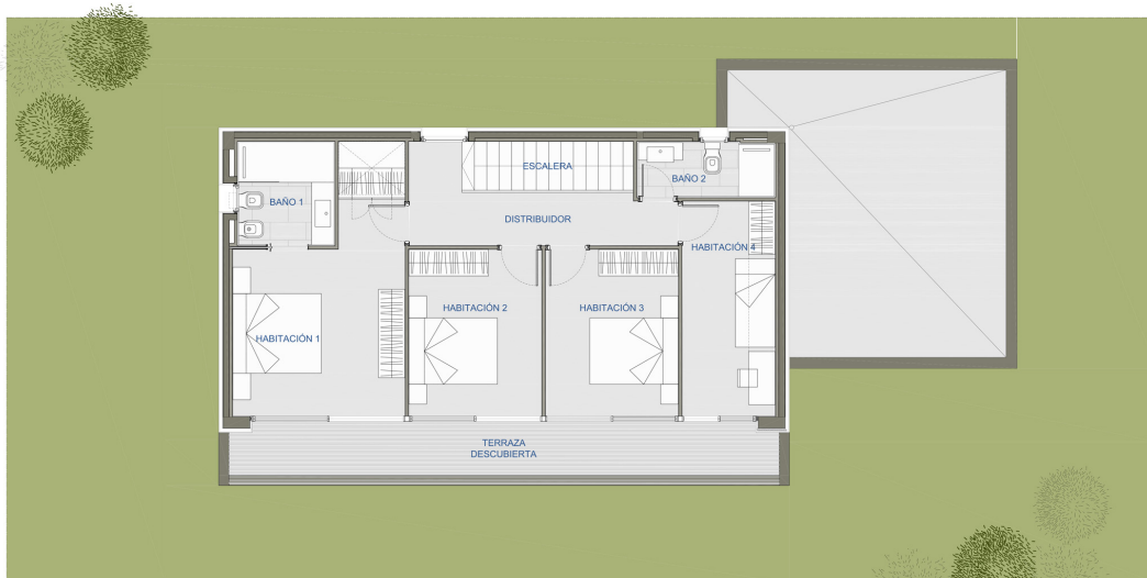
PLANTA PRIMERA
